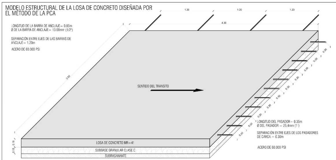
Ilustración 6. Esquema de la losa de pavimento de concreto (18 cm)
