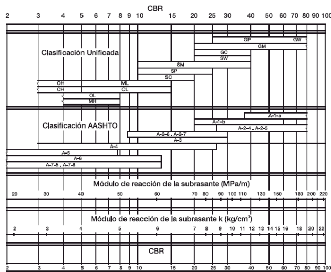
Ilustración 4. Correlación entre el CBR y el Módulo de Reacción
